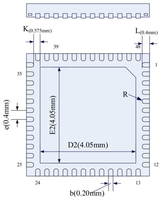
SK5301/SK5302/SK5305-LT 48-pin QFN (6x6x0.75mm)
