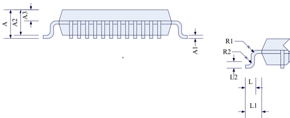
SK5301-LP 48-pin LQFP (7x7x1.6mm)
